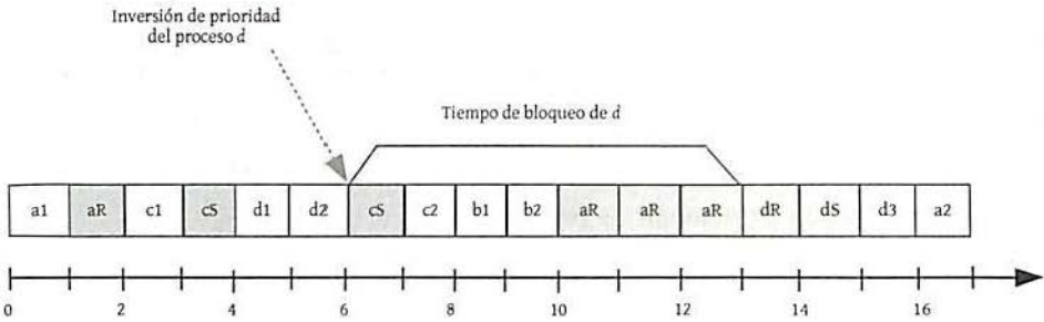
Figura 5.11: Diagrama de Gantt para el ejemplo de inversión de prioridad para el conjunto de procesos de la tabla 5.5.
