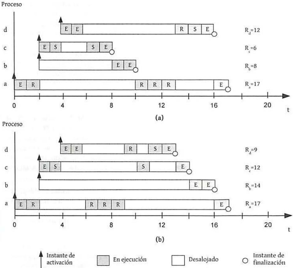
Figura 5.12: Líneas de tiempo para el conjunto de procesos de la tabla 5.5 utilizando a) un esquema de prioridades fijas con apropiación y b) el protocolo de herencia de prioridad. A la derecha de cada proceso se muestra el tiempo de respuesta asociado.
