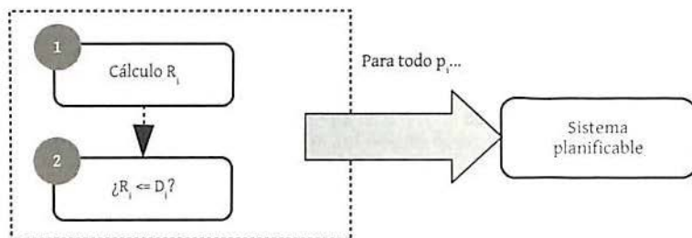
Figura 5.8: Esquema gráfico de un esquema de análisis del tiempo de respuesta para un conjunto de procesos o tareas.
