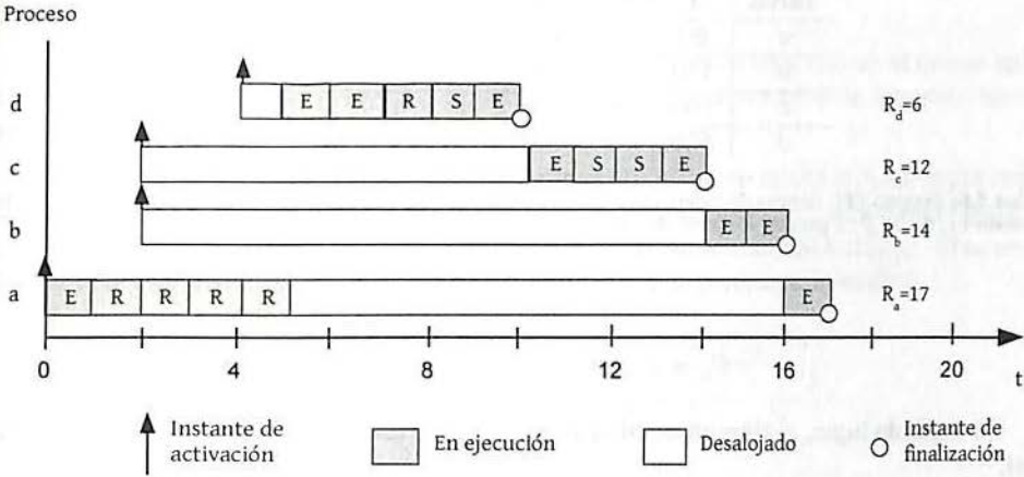
Figura 5.13: Línea de tiempo para el conjunto de procesos de la tabla 5.5 utilizando el protocolo de techo de prioridad inmediato.
