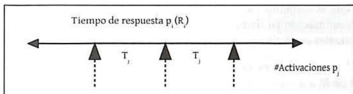
Figura 5.9: Esquema gráfica del número de activaciones de un proceso p_j con periodo T_j que interrumpe a un proceso p_i con un tiempo de respuesta total R_i .
